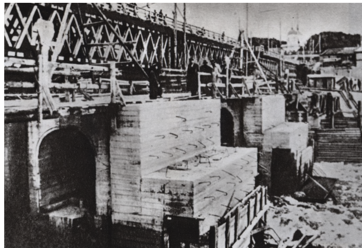
Dnjeprostroj Pamje e përgjithshme e digës, 1930
